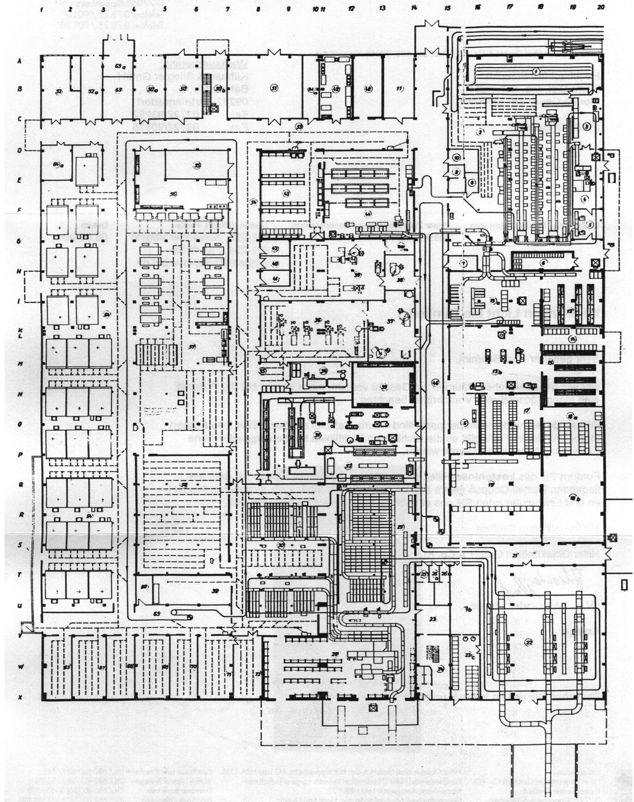
Grundriss Fleischverarbeitungsbetrieb mit Technologiebesatz
